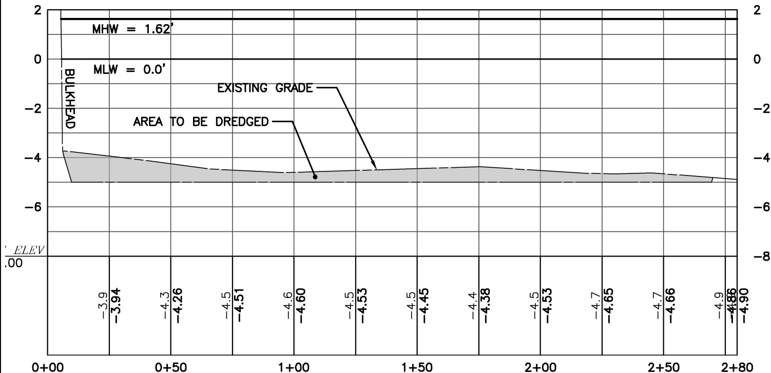
SECTION A HORIZONTAL SCALE: 1" = 40' VERTICAL SCALE: 1" = 4'
