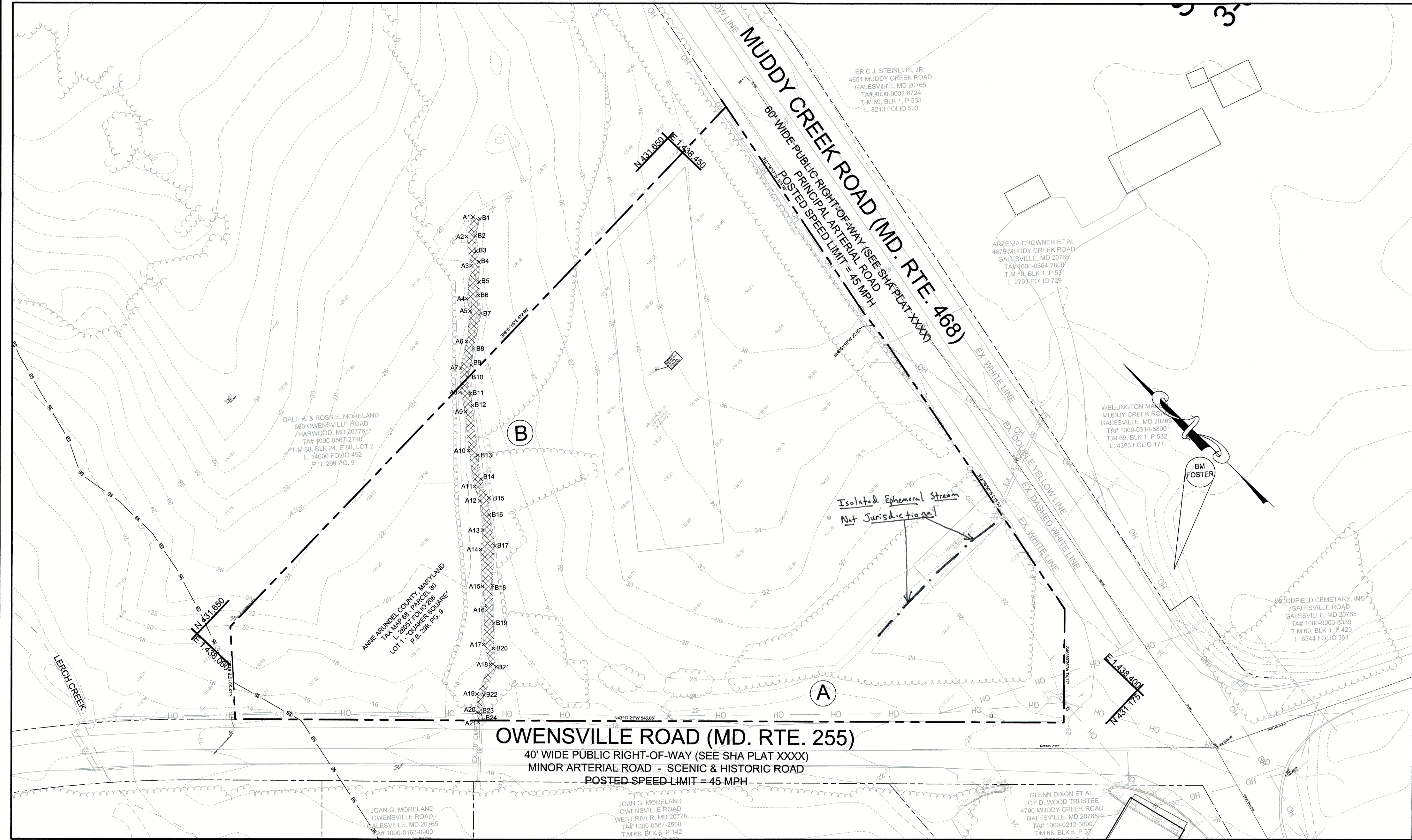
PLAN SCALE: 1" = 40'
